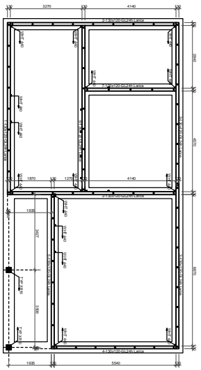
Pianta delle servitù Scala 1:50
