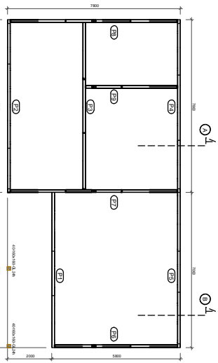
Pianta delle parti Scala 1:50
